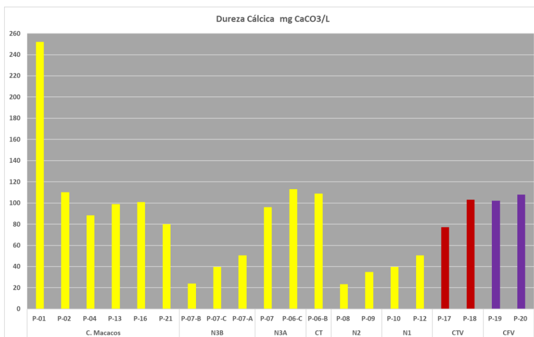
Figura 7.- Resultados do Biomonitoramento para o parâmetro Dureza Cálcica (mg CaCO 3 /L)
