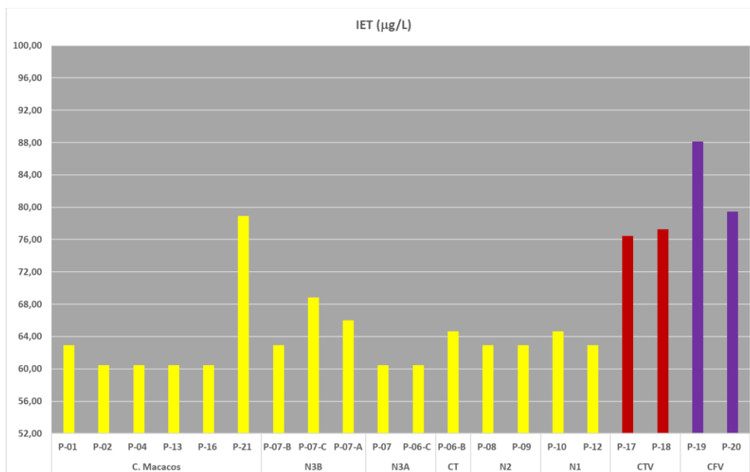
Figura 23.- Índice do Estado Trófico (IET) em \mu\text{g/L} para as amostras de água nos córregos em estudo do Projeto Izidora – 4ª campanha de Biomonitoramento – fevereiro 2023
