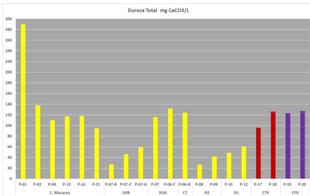
Figura 6.- Resultados do Biomonitoramento para o parâmetro Dureza Total (mg CaCO 3 /L)
